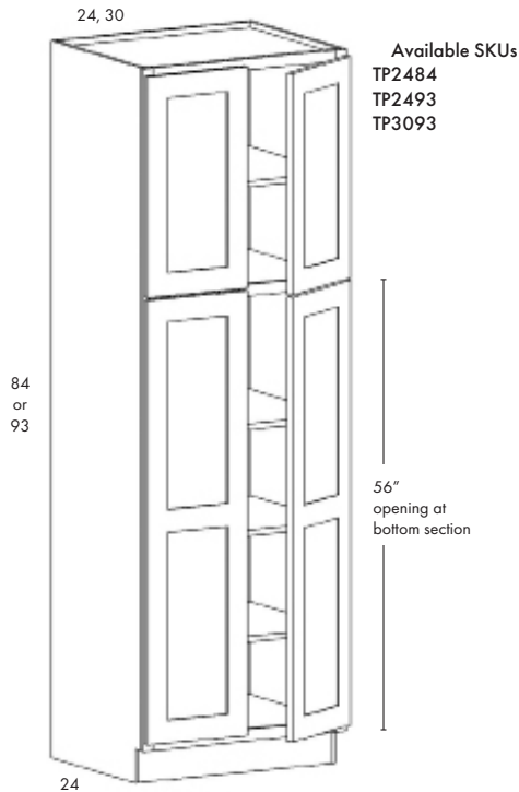
Paired Doors
